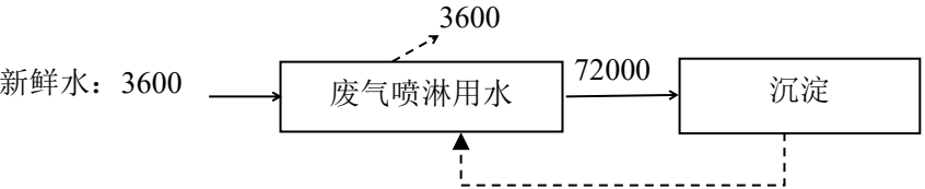
图 2-1 改建项目水平衡图（单位：m³/a）
