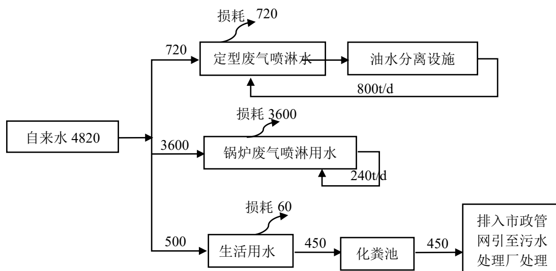
图 2-1 项目厂区水平衡图 (t/a)
