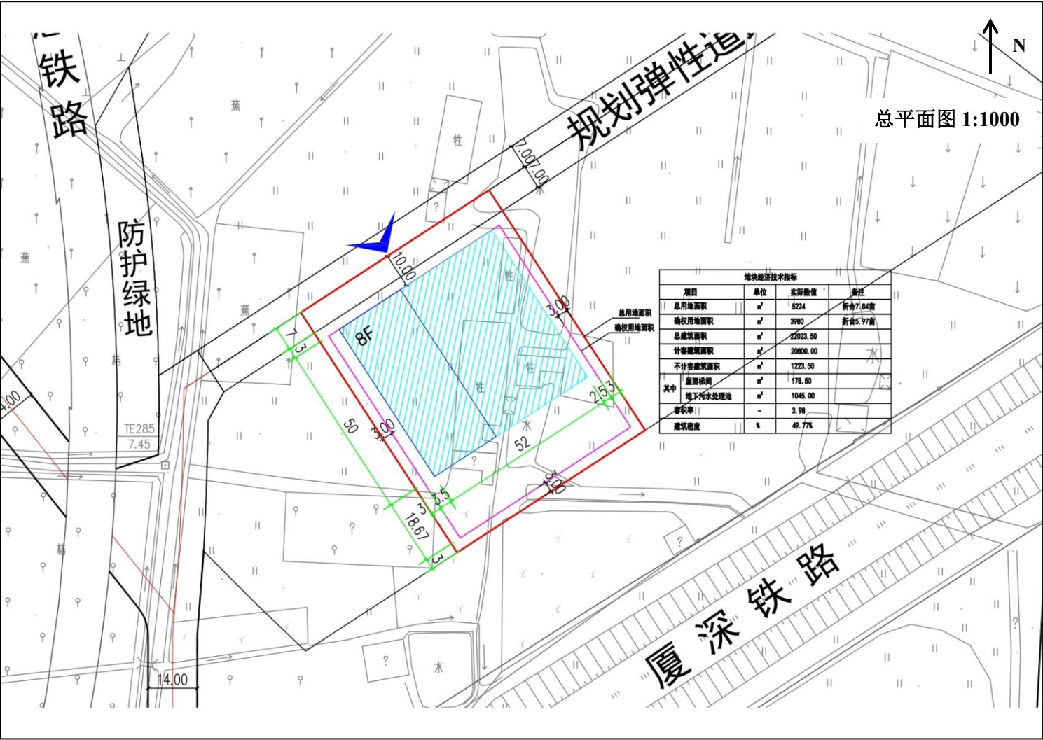
附图 5 总平面布置设计图
