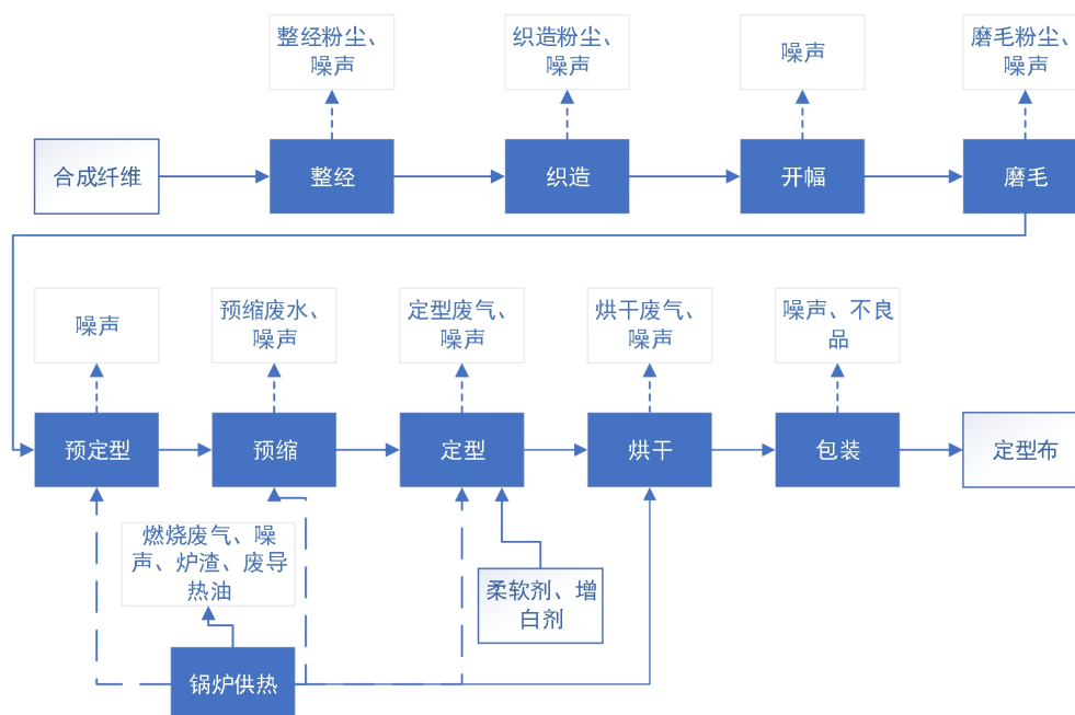
图2 工艺流程图
