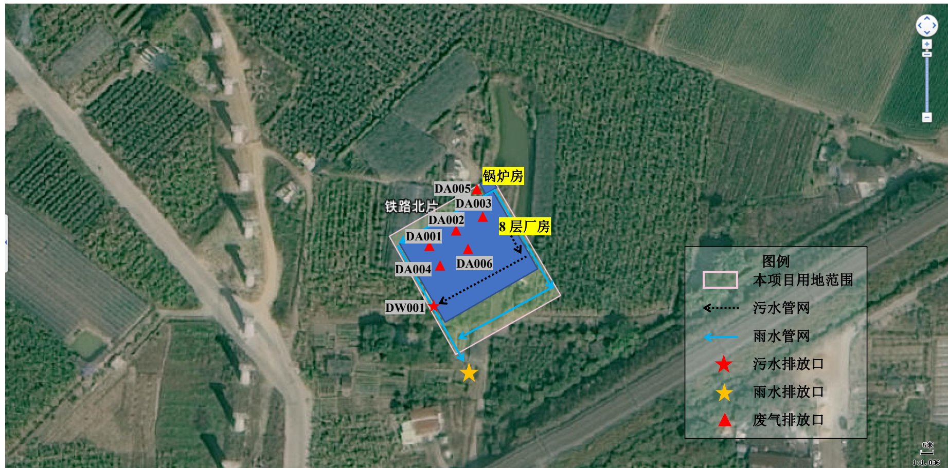
附图 6 总平面布置图
