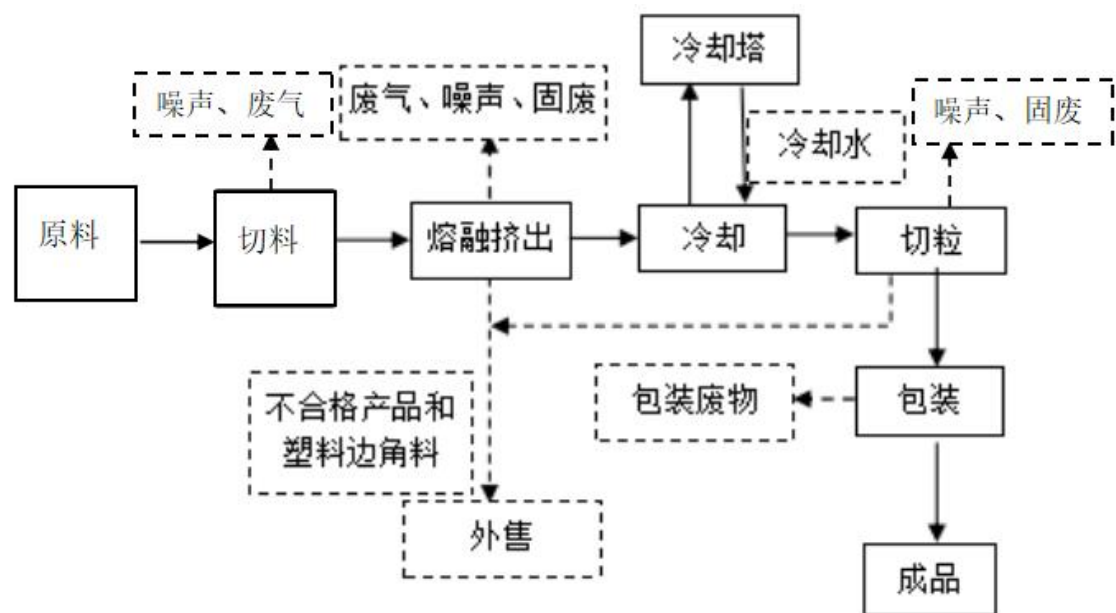
图 2-3 塑料粒生产工艺流程及产排污环节图
