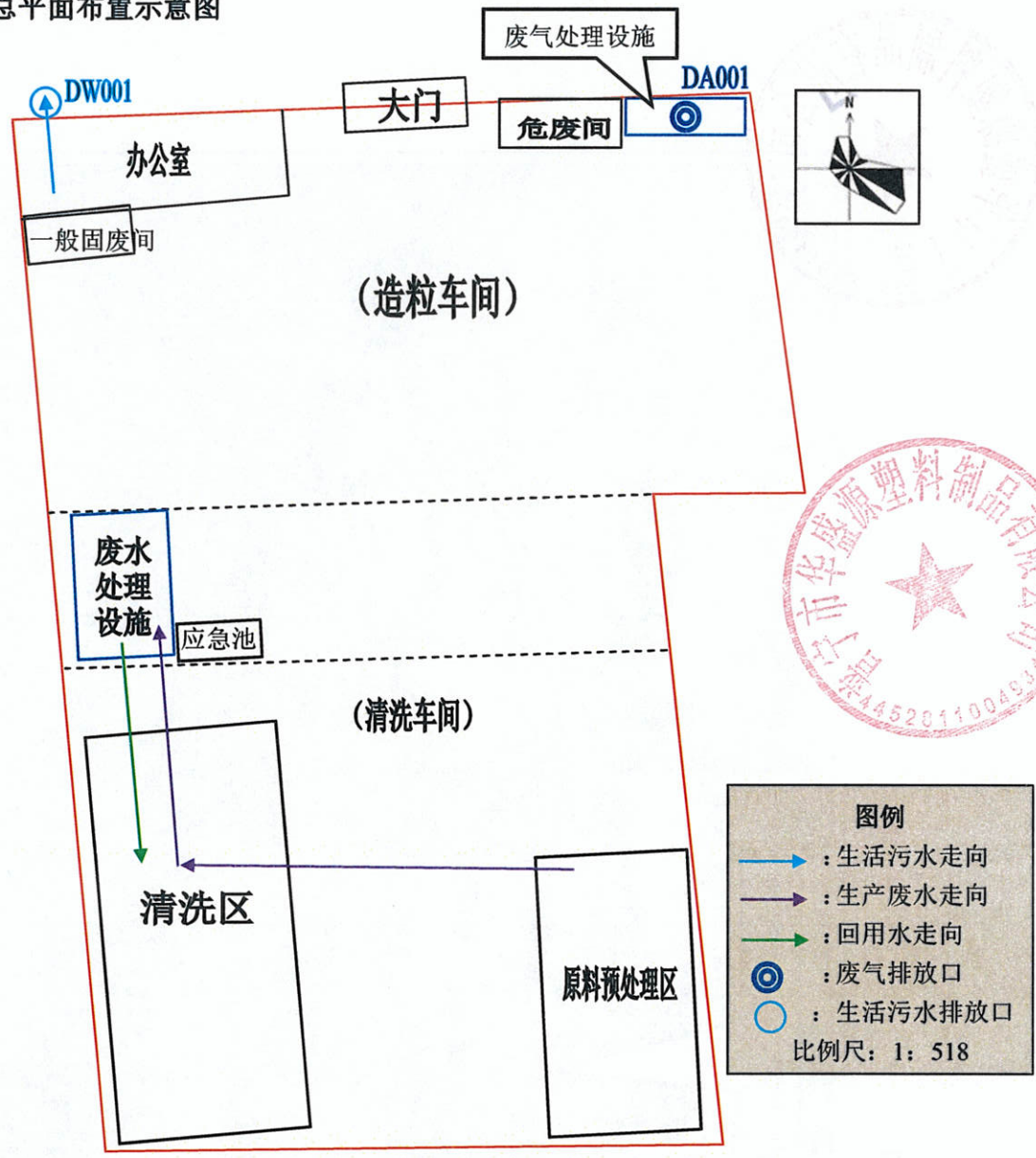
附图 5 项目总平面布置示意图
