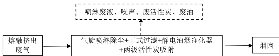
图 2-3 塑料粒生产工艺流程及产排污环节图
