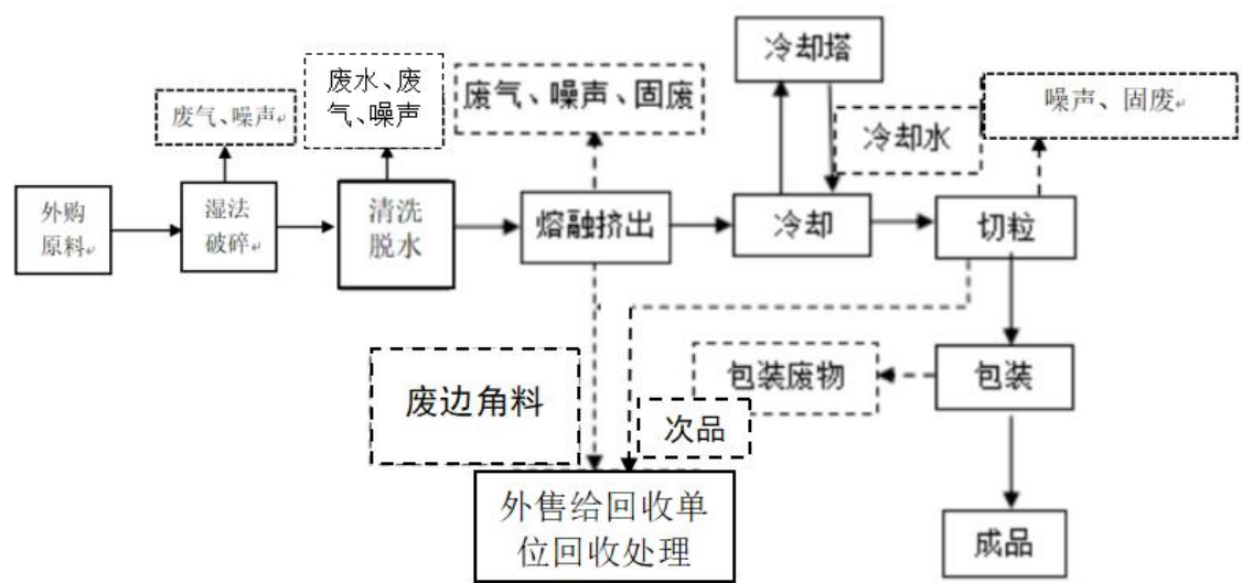
图 2-5 原项目生产工艺流程及产排污环节图
