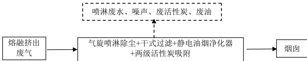
图 2-4 项目废气处理工艺流程及产污环节图
