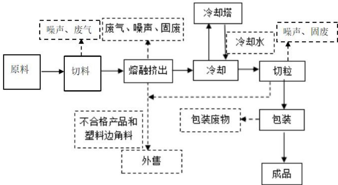
图 2-3 项目生产工艺流程及产排污环节图
