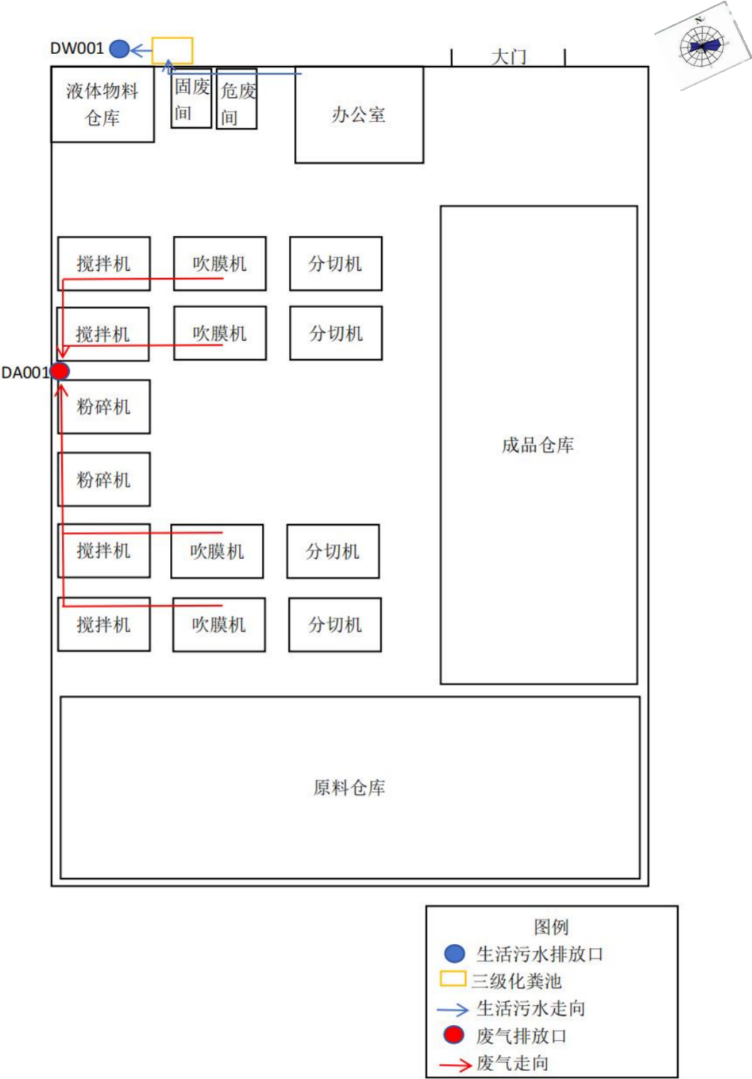
附图 10：平面布局图
