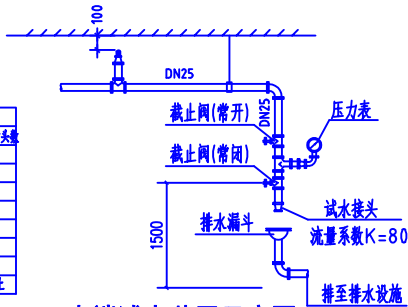
末端试水装置示意图
