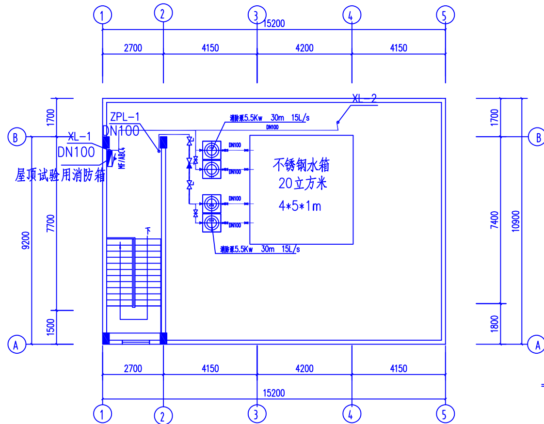
天面层消防供水布置图
