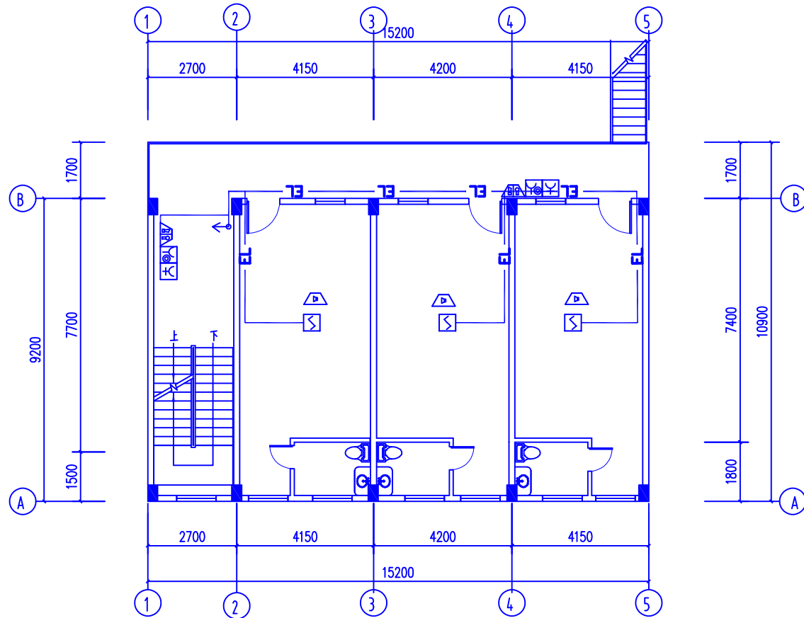
二层自动报警布置图
