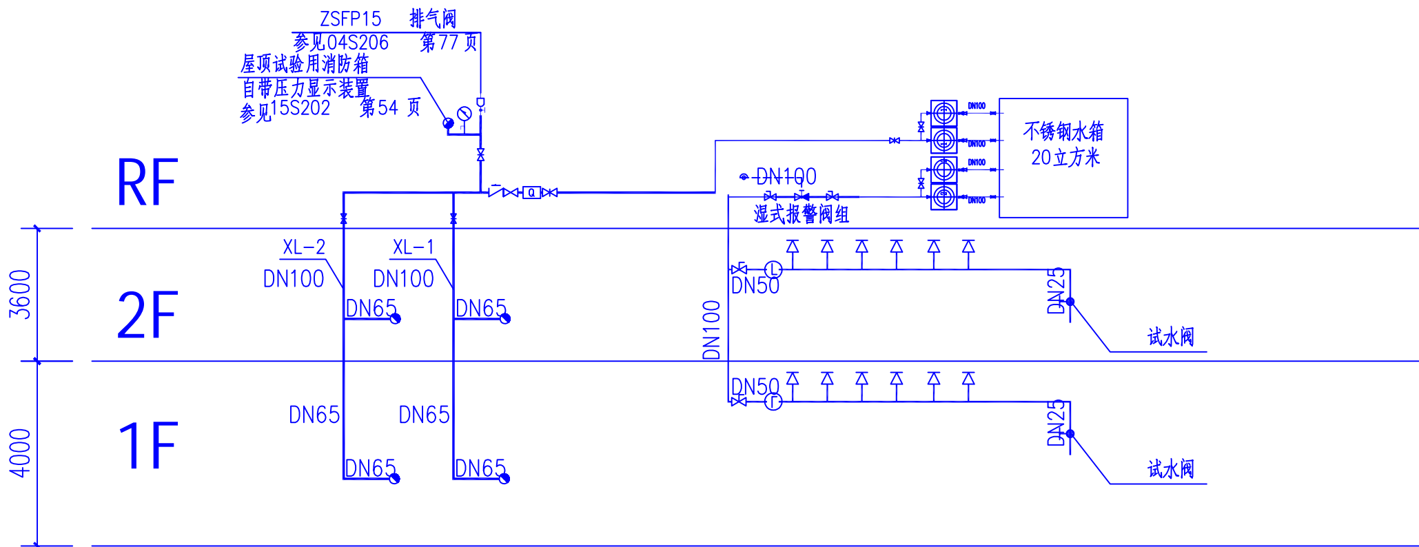
消火栓及喷淋系统图
