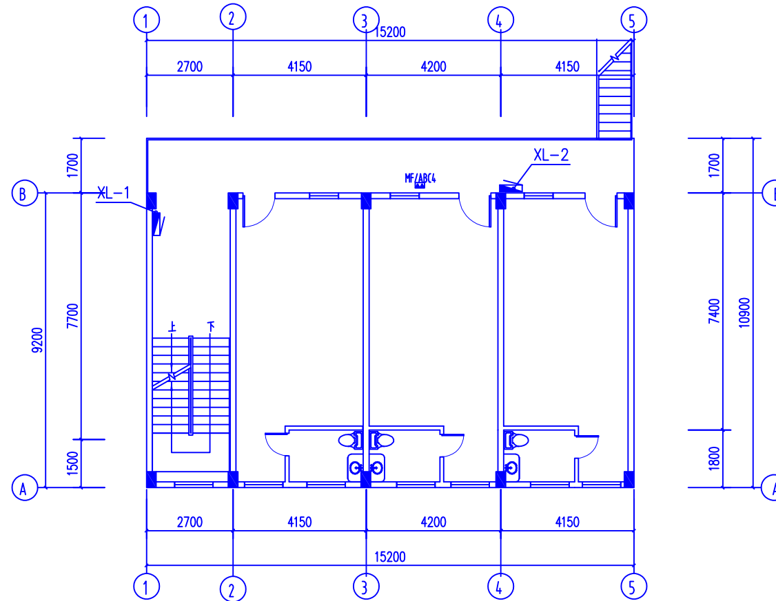
二层消火栓和灭火器布置图
