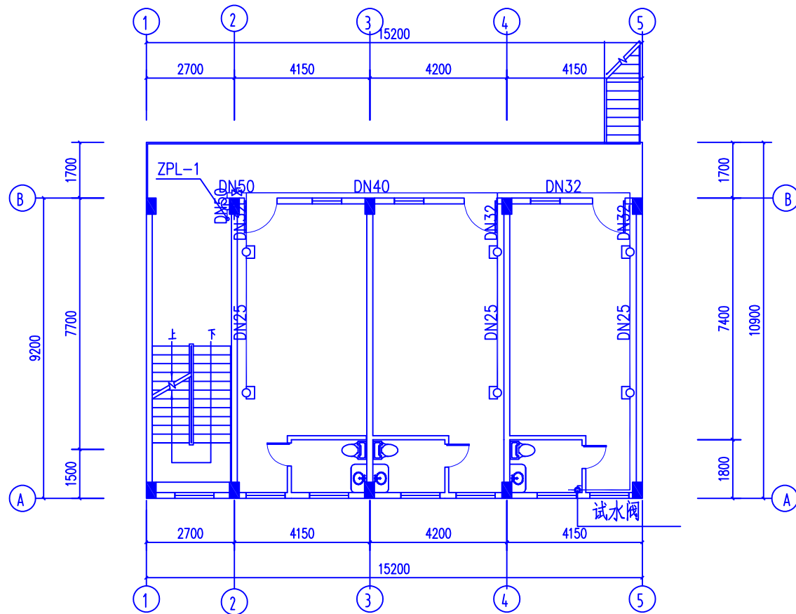
二层喷淋布置图
